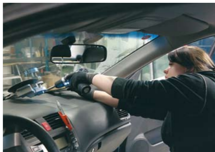
Liimanauhan alle ujutettavalla langalla leikataan liimapalko, jolloin saadaan tuulilasi irrotettua.
